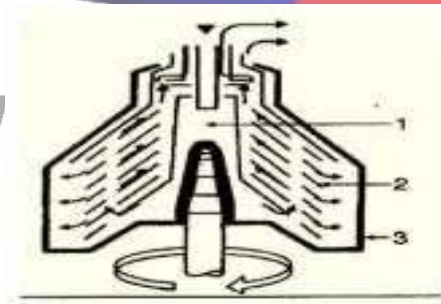
Gambar 8. Aliran dalam bowl purifier (sumber gambar. http://kapal-cargo.blogspot.com/2011/03/oil-purifier-kapal.html )
