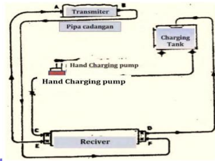
Gambar 32. Sistem pengisian ( charging system ) (sumber gambar. Suyanto, (1983) Pesawat Kapal, Pradnya Pramita)
