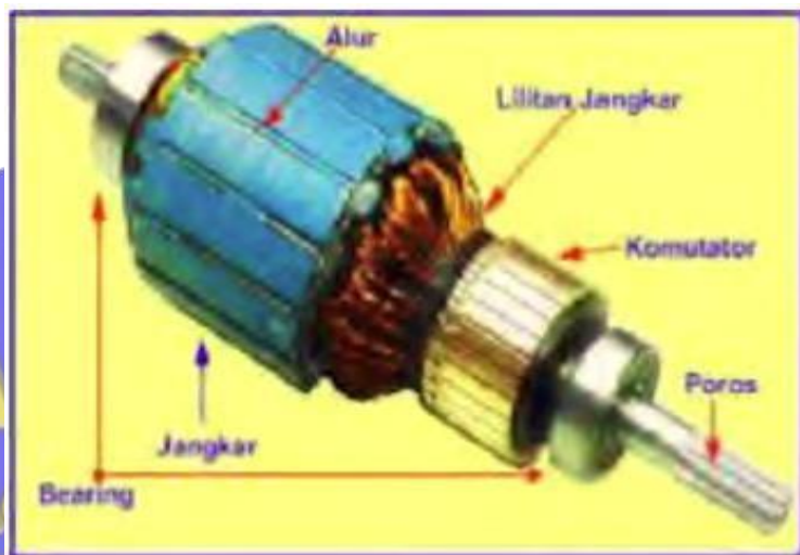
Gambar 37. Jangkar dengan lilitannya
