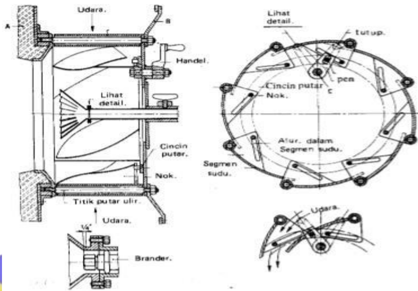
Gambar 24. Unit pengatur udara (sumber gambar. Suyanto, (1983) Pesawat Kapal, Pradnya Pramita)
