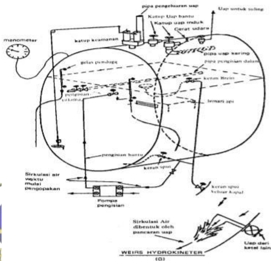
Gambar 17. Penempatan appendasi pada ketel Schots (sumber gambar. Suyanto, (1983) Pesawat Kapal, Pradnya Pramita)
