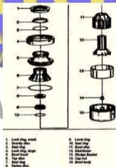
Gambar 10. Bagian dalam bowl (sumber gambar. http://kapal-cargo.blogspot.com/2011/03/oil-purifier-kapal.html )
