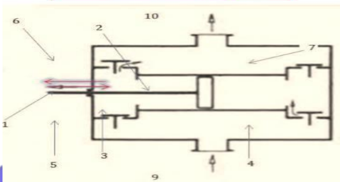
Gambar 39. Pompa torak kerja ganda
