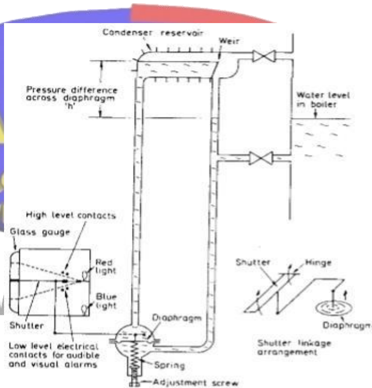
Gambar 20. Gelas penduga jarak jauh (sumber gambar. Suyanto, (1983) Pesawat Kapal, Pradnya Pramita)
