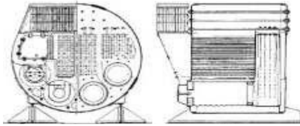
Gambar 13. Ketel Schot–jenis pipa api (sumber gambar. Suyanto, (1983) Pesawat Kapal, Pradnya Pramita)
