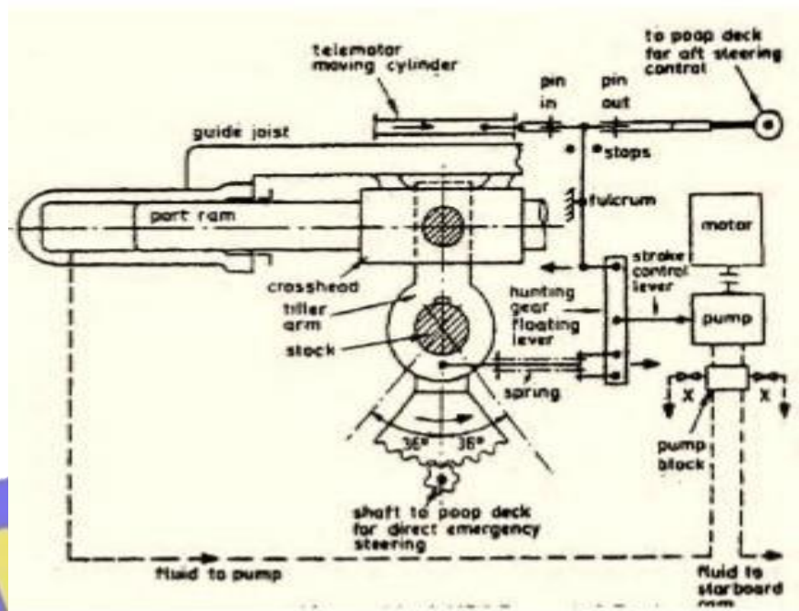
Gambar 26. Mesin kemudi hidraulik jenis 2 RAM (sumber gambar: Suyanto, (1983) Pesawat Kapal, Pradnya Pramita)
