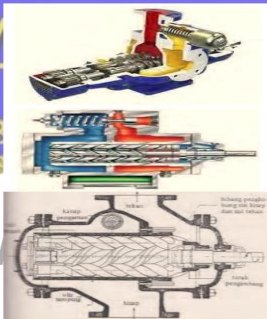
Gambar 48. Pompa I.M.O
