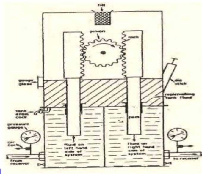
Gambar 30. Transmitter hidraulik (sumber gambar. Suyanto, (1983) Pesawat Kapal, Pradnya Pramita)
