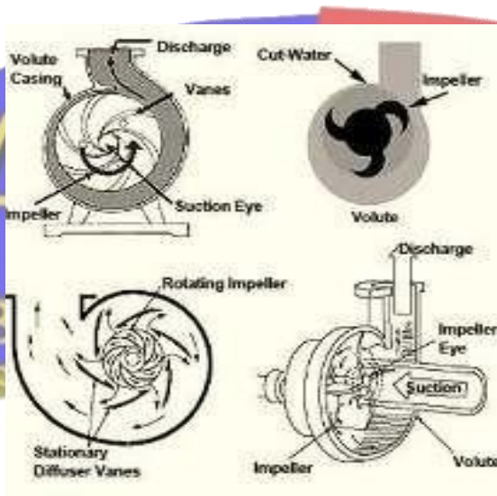
Gambar 43. Konstruksi pompa sentrifugal
