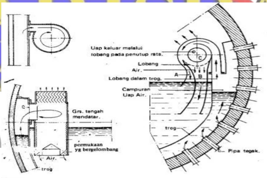
Gambar 22. Siklon horizontal
