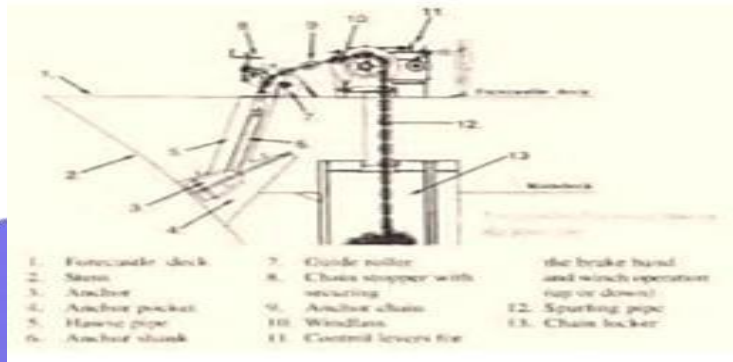
Gambar 33. Mesin penggulung jangkar
