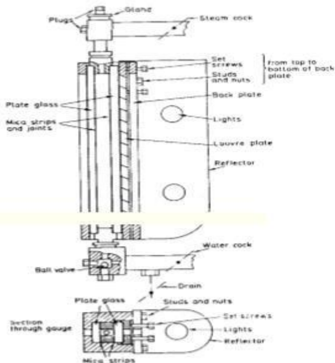
Gambar 19. Gelas penduga (sumber gambar. Suyanto, (1983) Pesawat Kapal, Pradnya Pramita)
