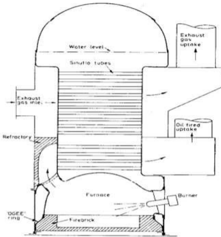
Gambar 16. Ketel bantu tegak
