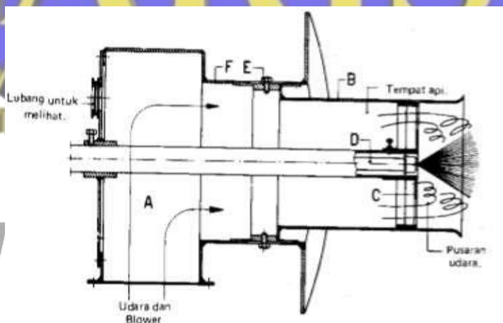
Gambar 23. Aliran udara untuk pembakaran
