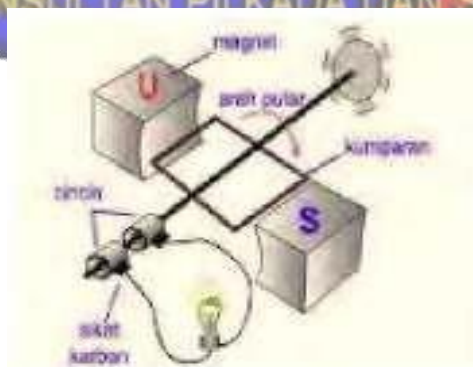
Gambar 36. Inti kutub magnet dan kumparannya
