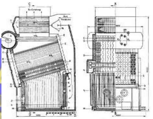
Gambar 14. Ketel B & W (sumber gambar. Suyanto, (1983) Pesawat Kapal, Pradnya Pramita)
