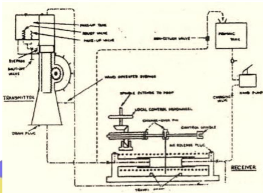
Gambar 29. Susunan unit telemotor (sumber gambar. Suyanto, (1983) Pesawat Kapal, Pradnya Pramita)
