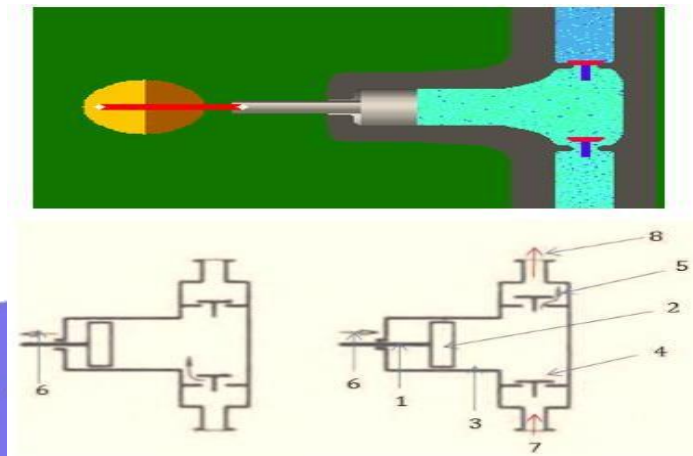
Gambar 38. Pompa torak kerja tunggal
