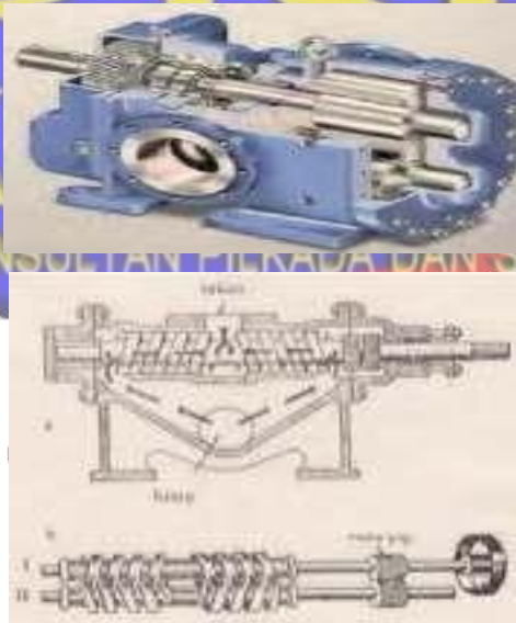
Gambar 47. Ulir Houttuin (sumber gambar. Suyanto, (1983) Pesawat Kapal, Pradnya Pramita)
