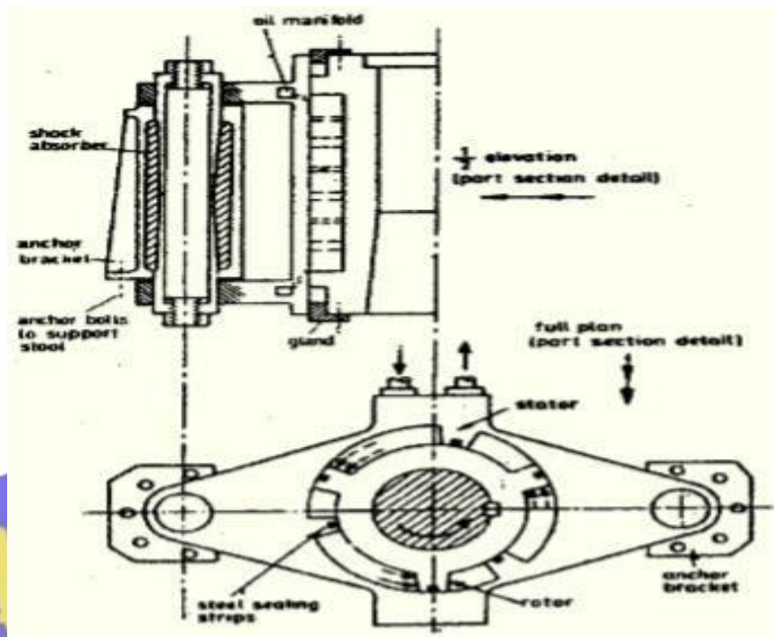
Gambar 27. Mesin kemudi jenis vane rotary (sumber gambar. Suyanto, (1983) Pesawat Kapal, Pradnya Pramita)
