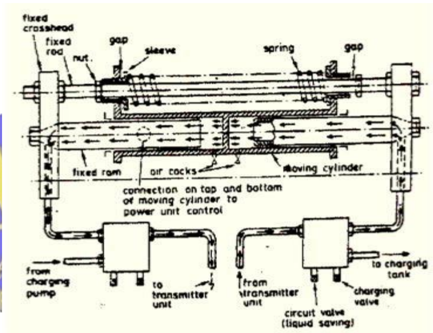
Gambar 31. Receiver hidrolik (sumber gambar. Suyanto, (1983) Pesawat Kapal, Pradnya Pramita)
