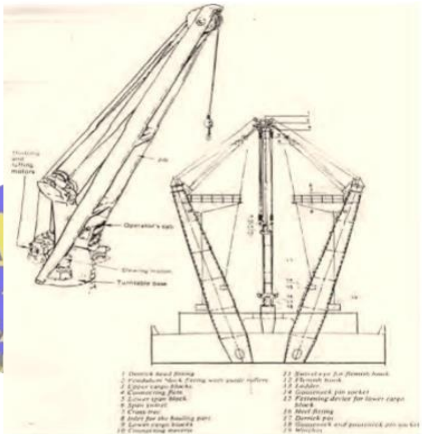
Gambar 34. Derek kapal
