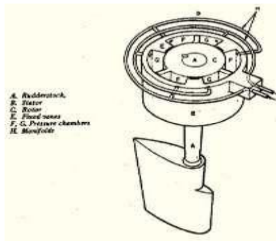
Gambar 28. Bagian-bagian mesin kemudi jenis vane rotary (sumber gambar. Suyanto, (1983) Pesawat Kapal, Pradnya Pramita)
