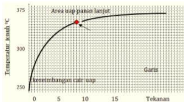
Gambar 12. Keseimbangan tekanan dan temperatur (sumber gambar. Suyanto, (1983) Pesawat Kapal, Pradnya Pramita)
