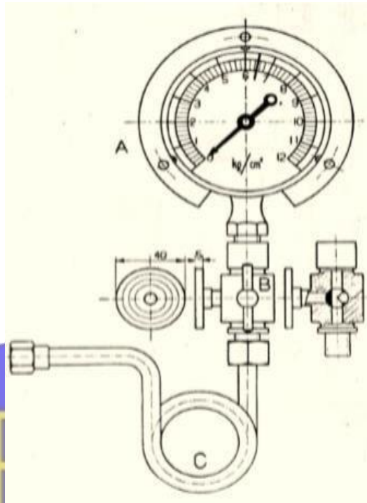
Gambar 18. Manometer untuk ketel uap (sumber gambar. Suyanto, (1983) Pesawat Kapal, Pradnya Pramita)
