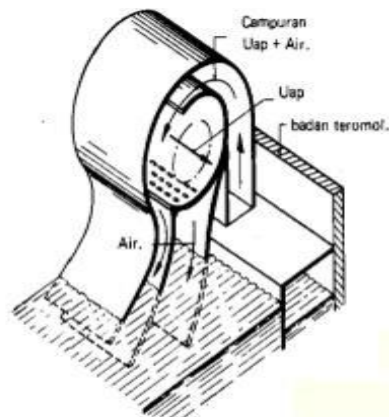
Gambar 21. Siklon horizontal
