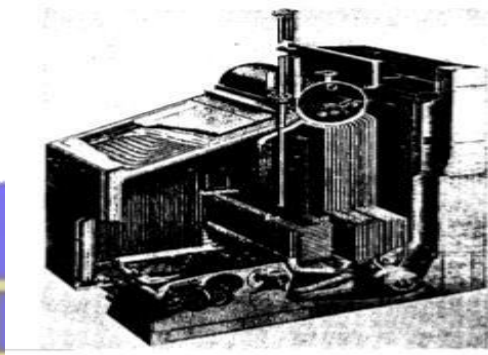
Gambar 15. Ketel B & W jenis lain (sumber gambar. Suyanto, (1983) Pesawat Kapal, Pradnya Pramita)
